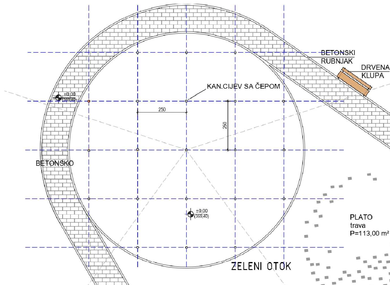
slika 9. Prikaz dispozicije procjednica oborinske odvodnje
