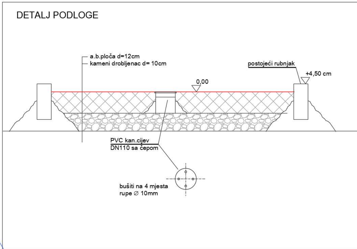
slika 10. Presjek podloge
