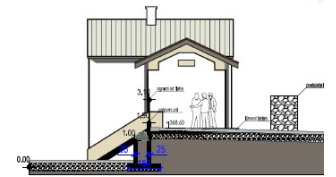
PRESJEK - POGLED D-D'
