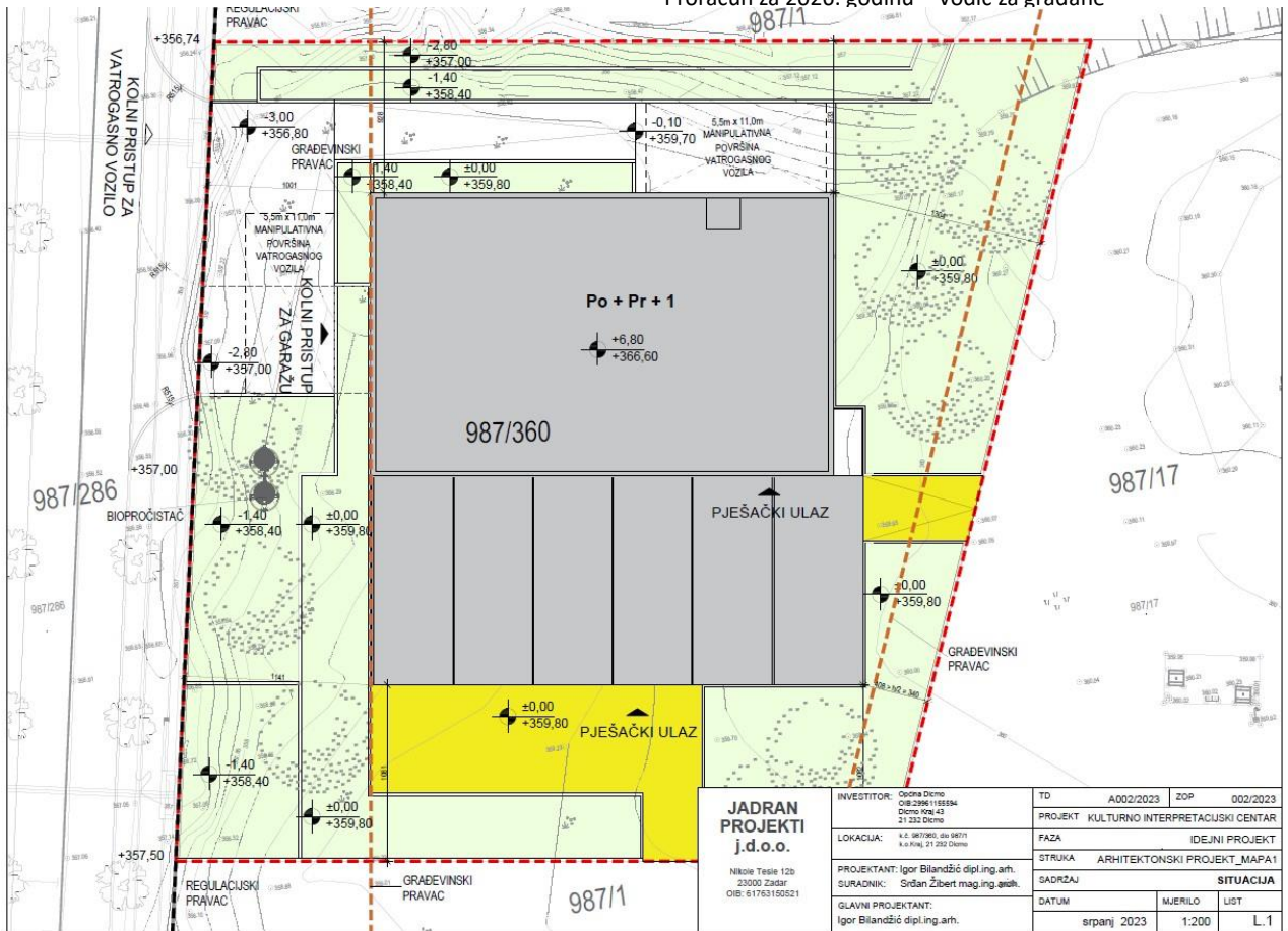
Kulturno interpretacijski centar Dicmo – Idejni projekt
